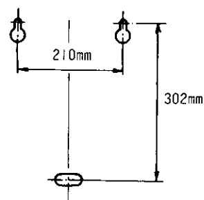
取り付け寸法図
